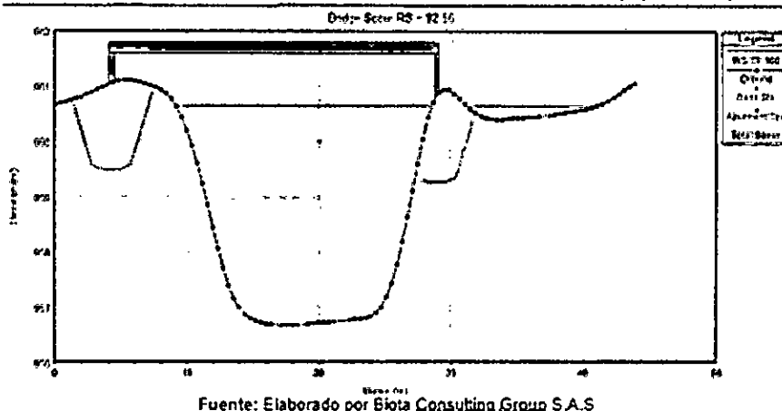
Figura 7-2. Socavación local en condiciones existentes para El río Villa Vieja (K0+190,39)
