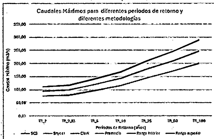
Figura 9-1 Variación de caudales máx. vs. T_R condición AMCH (D) – El río Vito Vieja a la altura de las coordenadas 4.776.176,70339 m Este y 1.895.170,32138 m Norte
