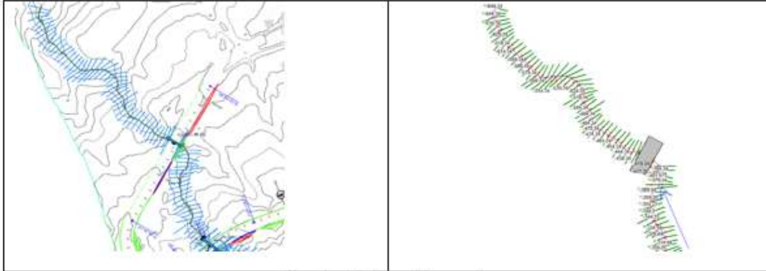
Figura 21. Distribución de las secciones transversales proyectadas
