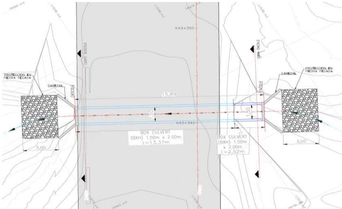
Figura No. 3. Esquema de obra Hidráulica Propuesta UF2 – ID-364 abscisa de diseño K42+343.
