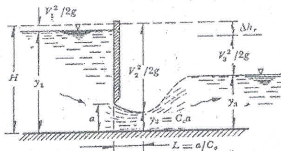
Ilustración 1. Detalle de Compuerta deslizante.
