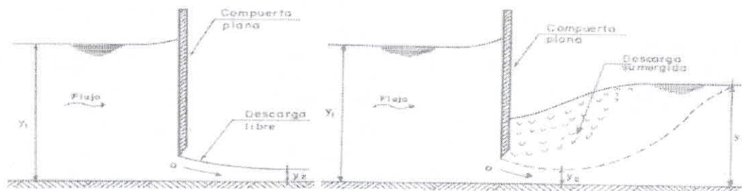
Ilustración 2. Tipo de descarga en compuertas.
