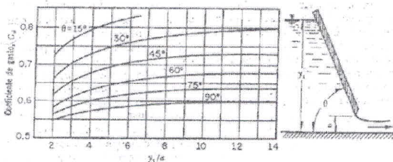
Ilustración 6. Coeficiente de gastos para las compuertas planas inclinadas con descarga libre. Fuente: Redicado CAM-18959
