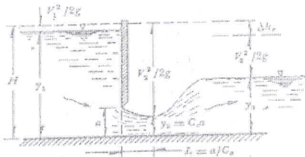
Ilustración 1. Detalle de Compuerta deslizable.
