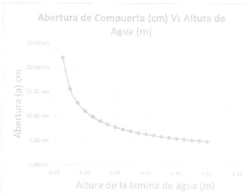
Ilustración 10. Valores de diseño de la regleta graduada con las aberturas correspondientes, acordes a la lámina de agua. Fuente: Radicado CAM-18959
