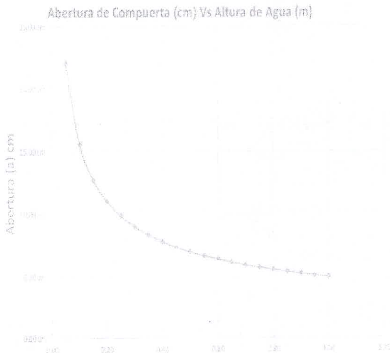
Ilustración 13. Valores de diseño de la regla graduada con las aberturas correspondientes acordes a la lámina de agua. Fuente. Radicado CAM-18959
