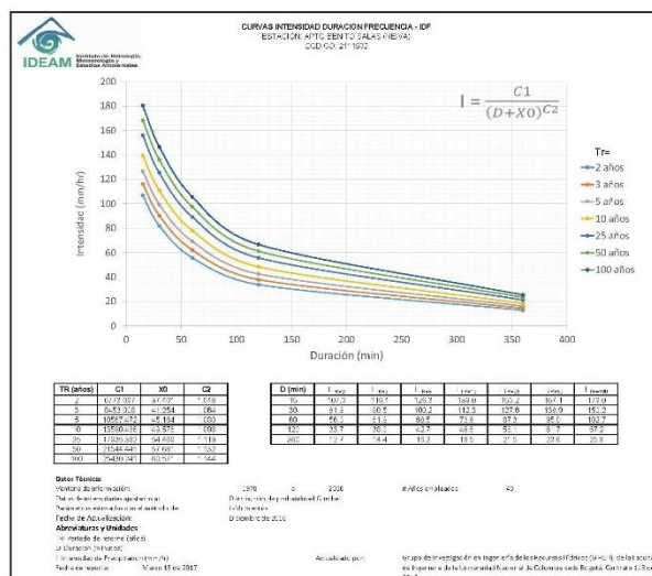
Gráfico 12. CURVAS IDF
