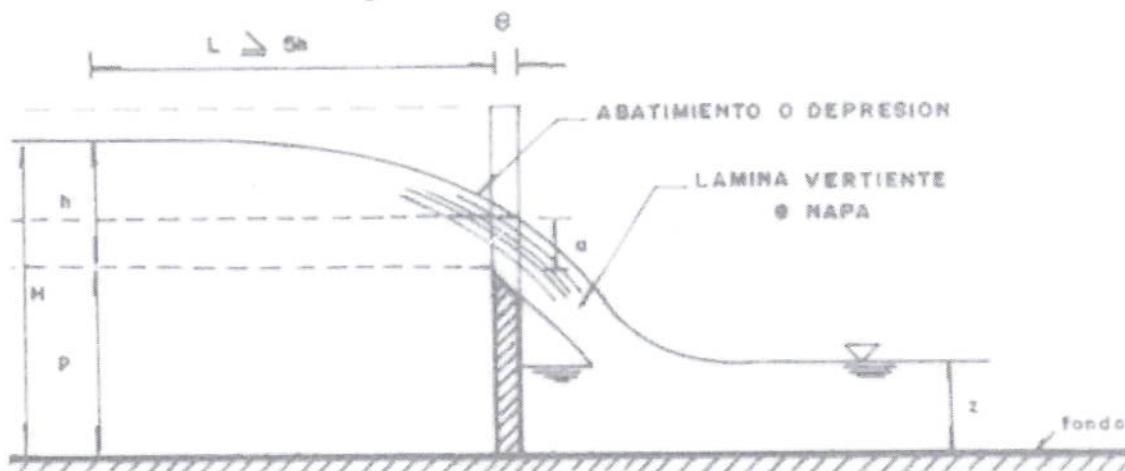
Figura 9 Localización Limnómetro
