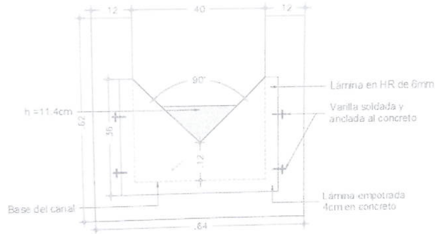
Figura 7 Vertedero Triangular de Pared Delgada
