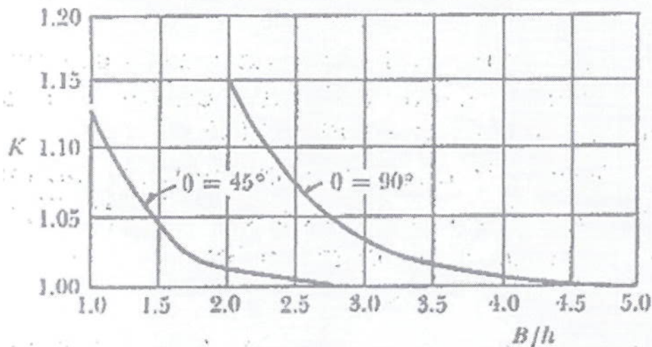
Figura 5 Valores de K para la fórmula de la Universidad Católica
