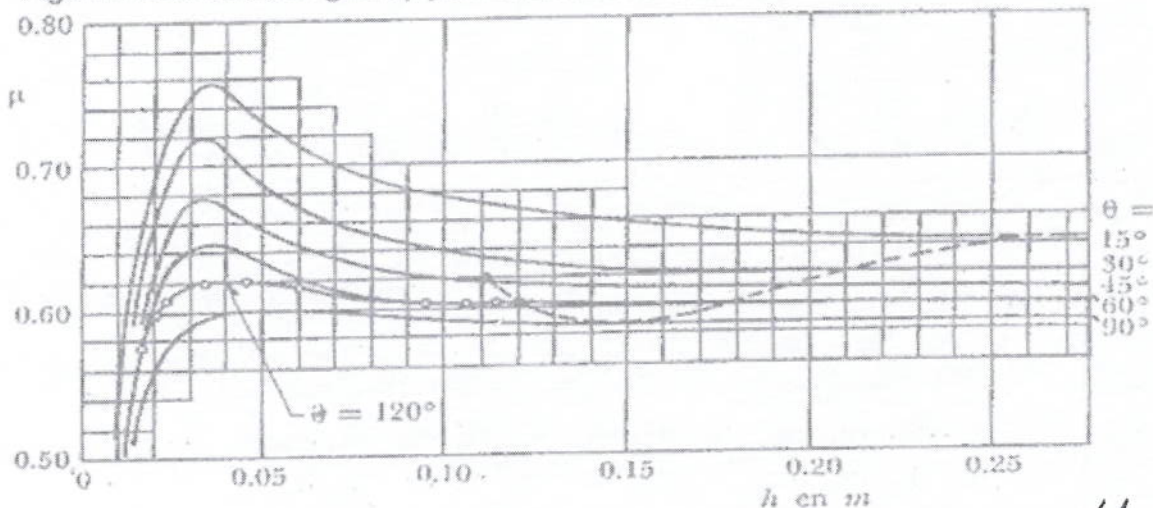
Figura 4 Coeficiente de gasto \mu para la fórmula de la Universidad Católica de Chile
