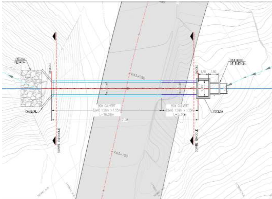
Figura No. 3. Esquema de obra Hidráulica Propuesta UF2 – ID-367 abscisa de diseño K43+091.
