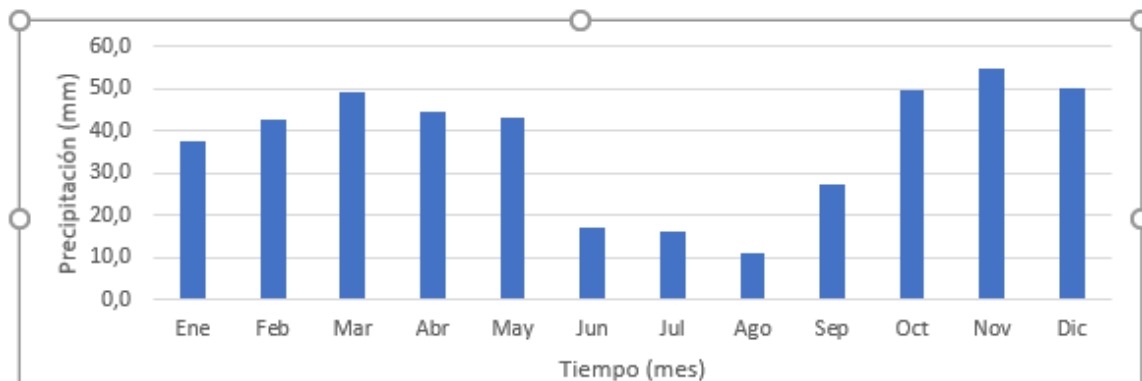
Figura 16. Precipitación máxima en 24 horas mensual
