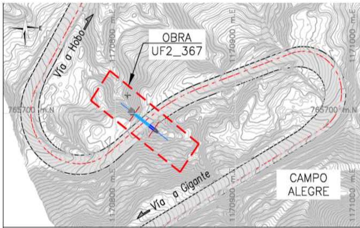
Fotografía 1, 2 y 3. Obra hidráulica existente UF2-ID- 367 ubicada en la abscisa de diseño K43+091 (encole).
