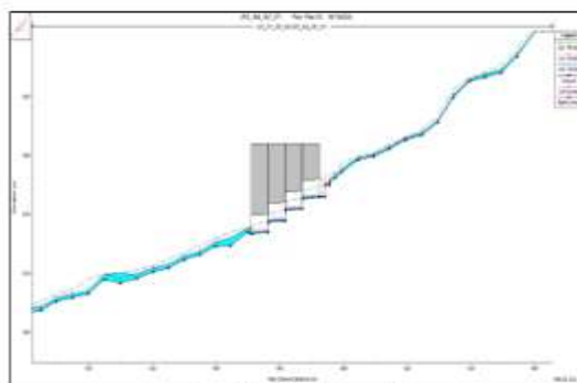
Figura 26. Perfil lámina de agua obra proyectada, TR 100 años
