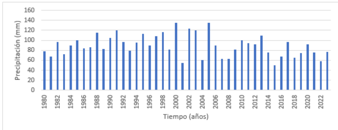
Figura 15. Precipitación máxima en 24 horas multianual
