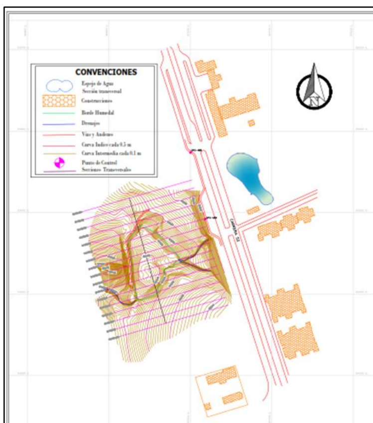
Figura 18. Curvas a nivel cada 10 centímetros humedal El Curíbano
