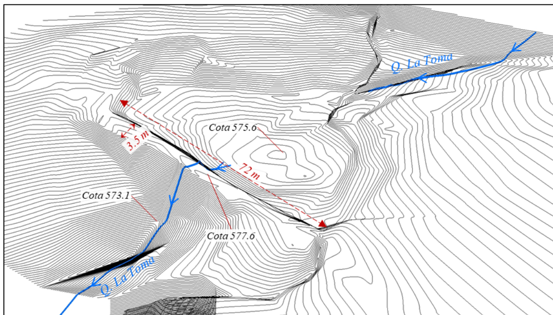
Figura 99. Levantamiento topográfico y batimétrico Humedal Curíbano
