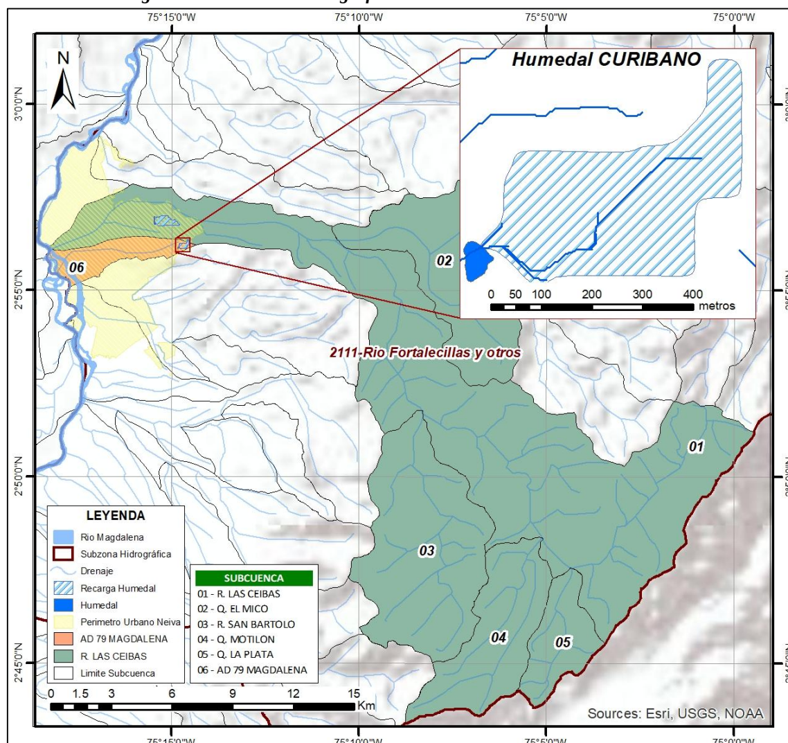
Figura 19. Subcuenca hidrográfica asociada al Humedal Curibano
