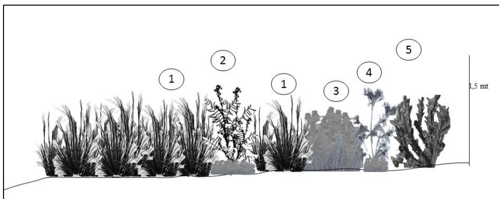
Figura 42. Perfil de vegetación transecto 3.
