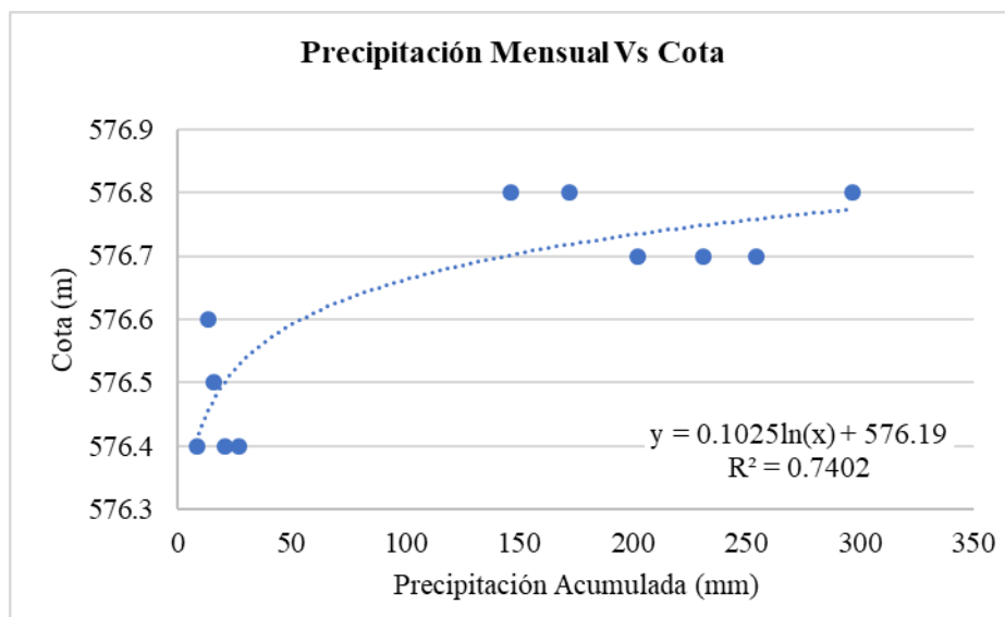
Figura 104. Precipitación acumulada mensual versus altura – Humedal El Curíbano
