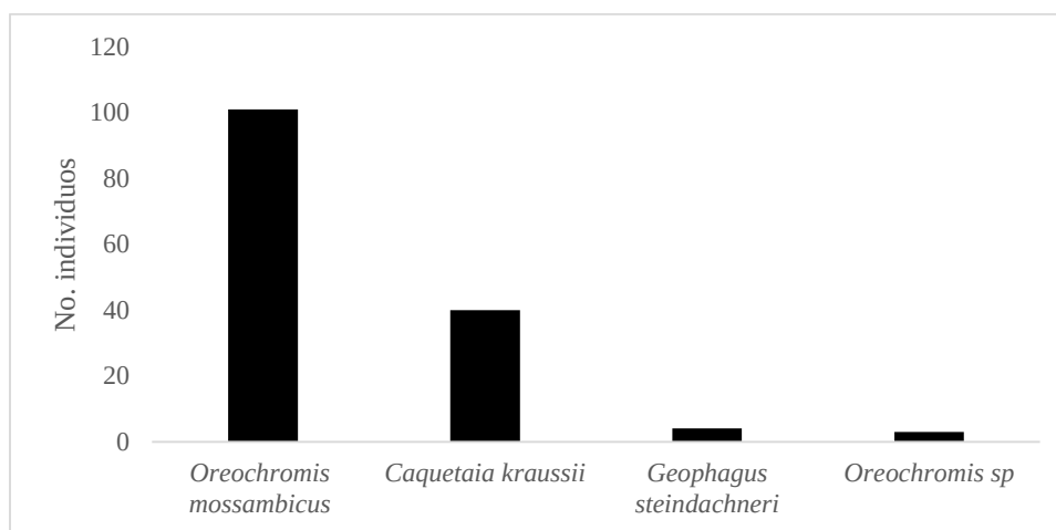
Figura 87. Abundancia de las especies de peces registradas en humedal El Curíbano
