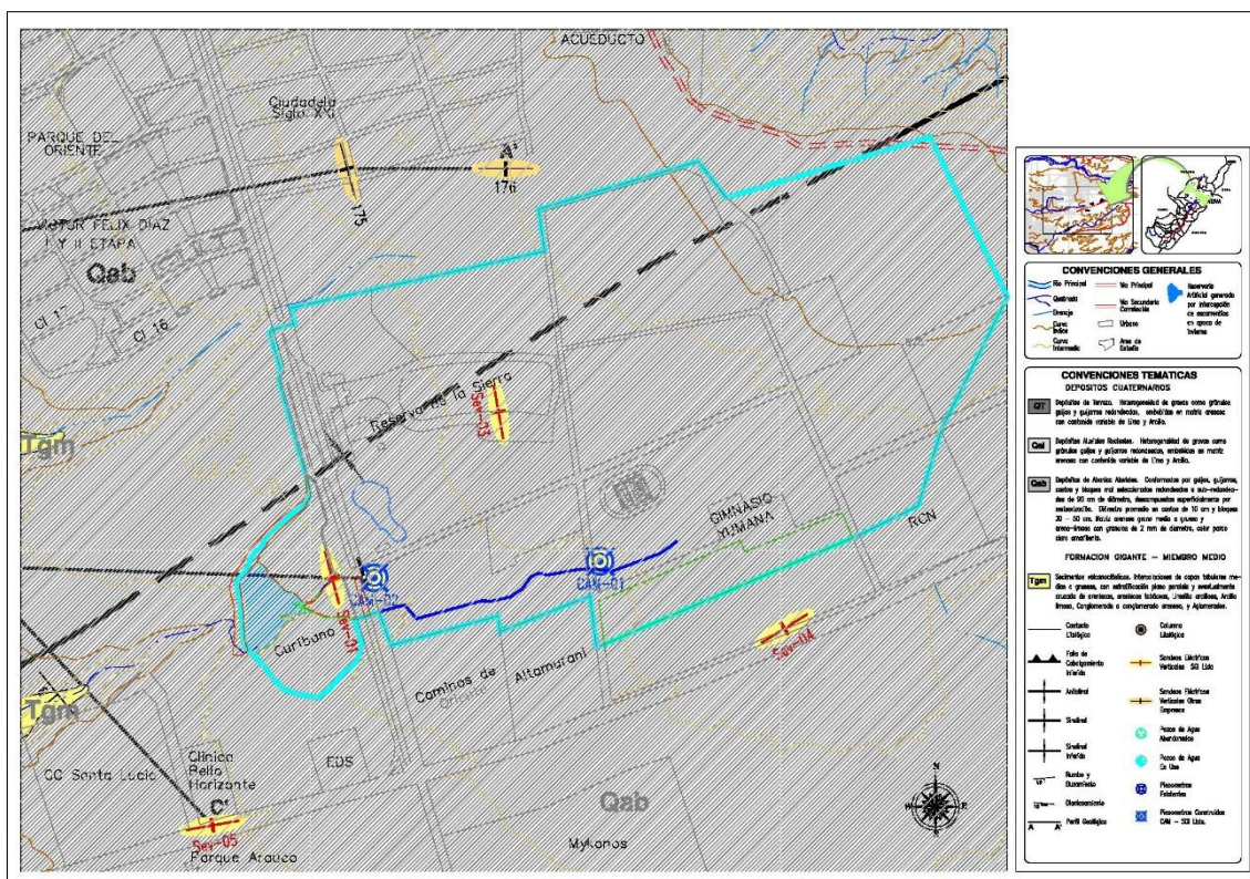
Figura 22. Mapa geológico de la zona del humedal
