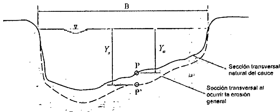
Figura 23. Esquema de descenso del lecho por socavación general
