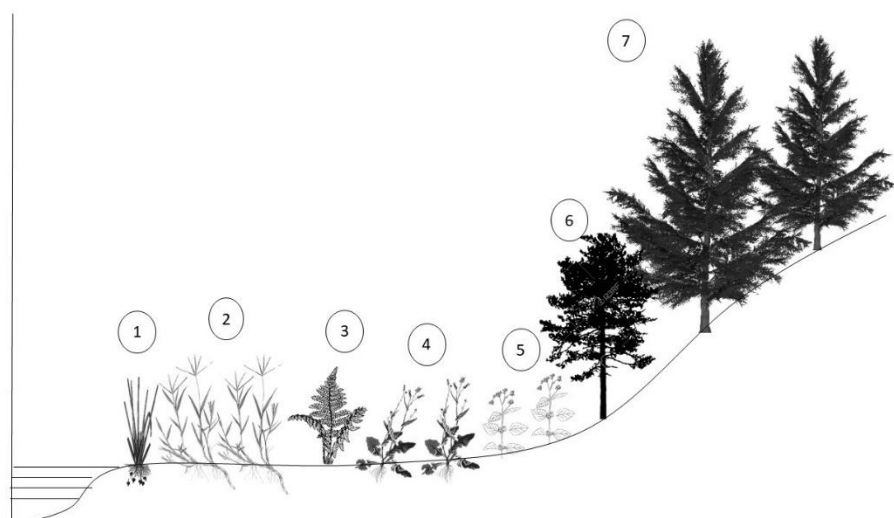
Ilustración 3. Perfil de vegetación transecto No. 3. Especies: 1 Eleocharis geniculata ; 2. Cynodon dactylon ; 3. Osmunda regalis ; 4. Emilia sonchifolia ; 5. Sida rhombifolia ; 6. Palicourea guianensis ; 7. Pinus patula .
