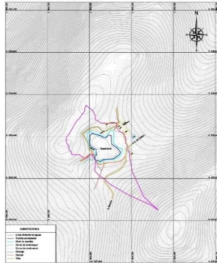
Figura 10. Levantamiento altiplanimétrico del humedal
