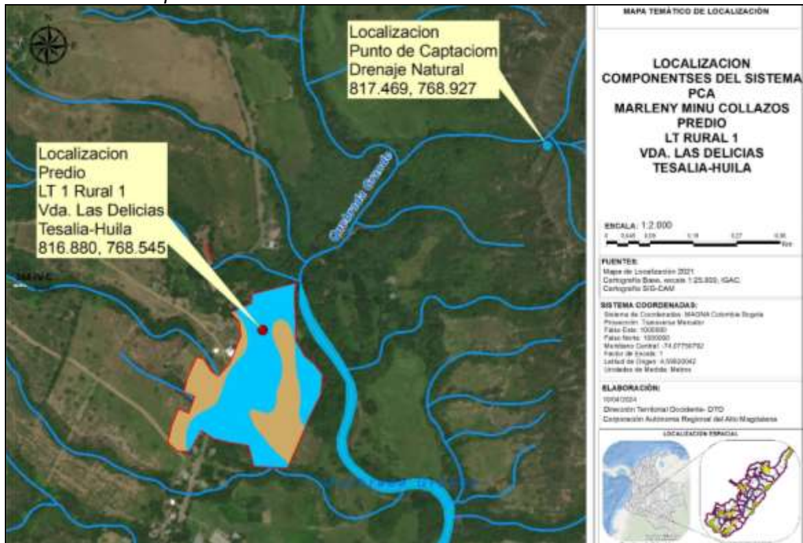
Figura 19 Localización Componentes Del Sistema.
