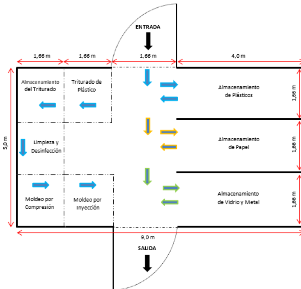
Figura 3. Plano de la caseta ambiental propuesta
