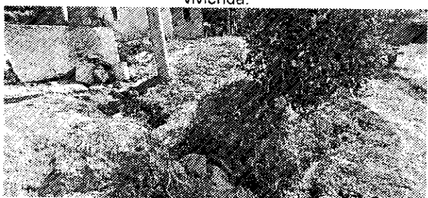
Fotografía 4. Zanja de conducción de aguas grises
