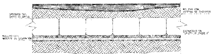
Figura ¡Error! No hay texto con el estilo especificado en el documento.-1. Detalle Constructivo Cruce Subfluvial
