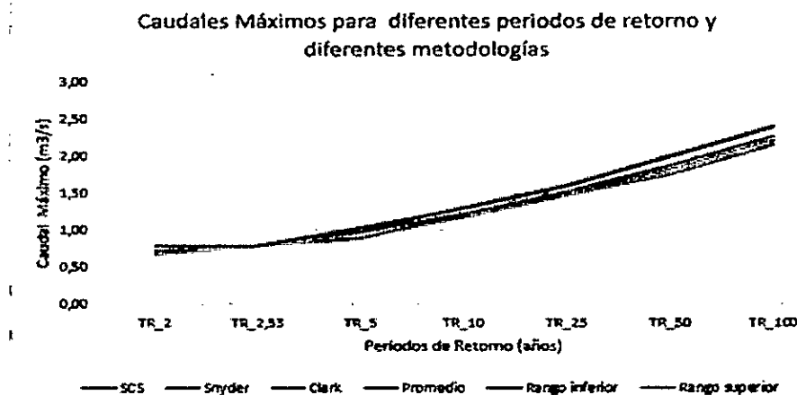
Figura 9-1 Variación de caudales máx. vs. T, condición AMCII (B) –La quebrada "Paso Quebrada"
