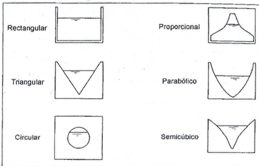
Figura 1 Formas de vertedero
