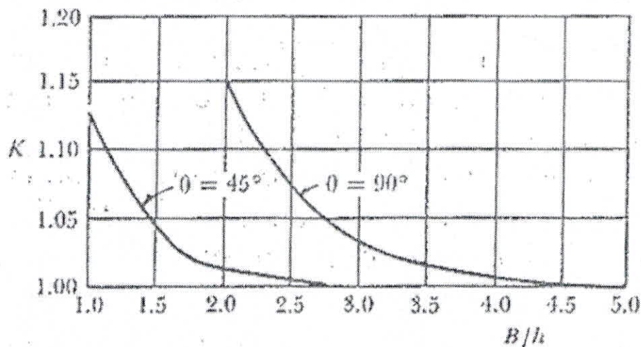
Figura 5 Valores de K para la fórmula de la Universidad Católica
