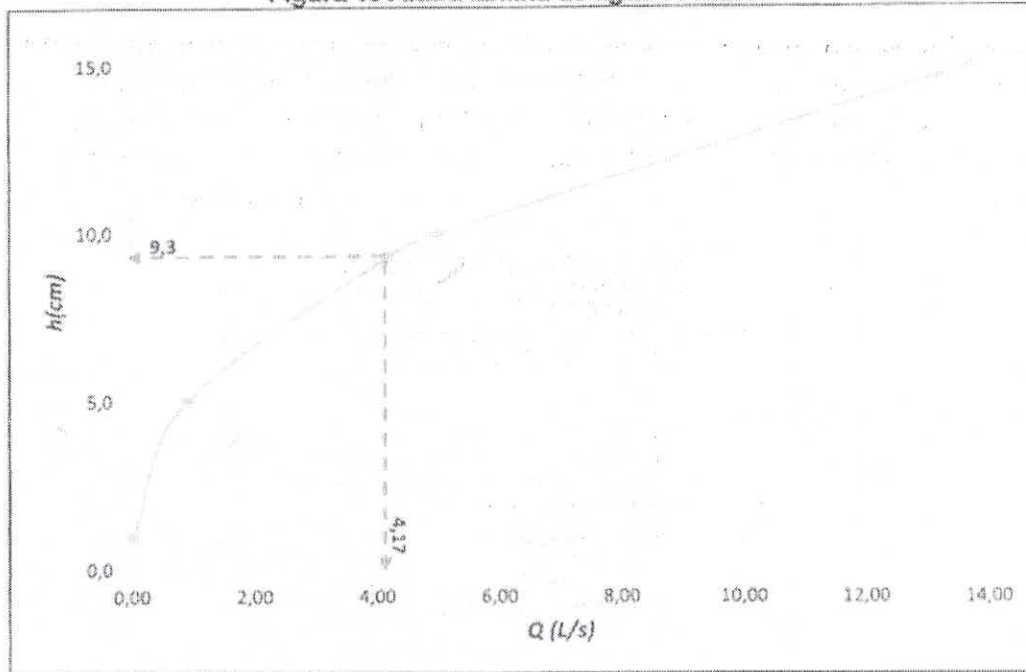
Figura 10 Altura lámina de agua vs caudal
