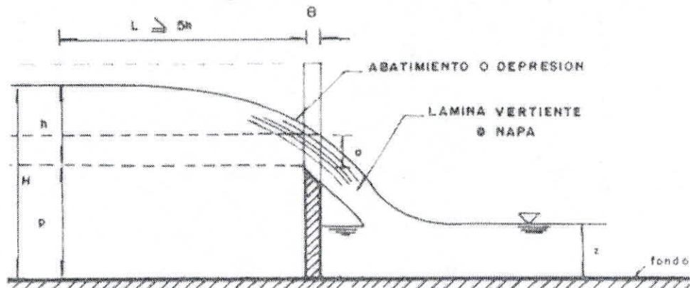
Figura 9 Localización Limnómetro
