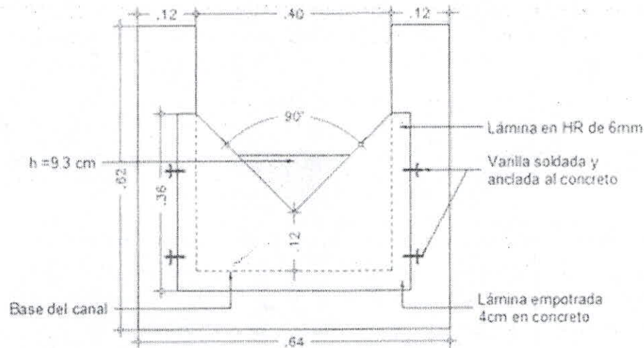
Figura 8 Vertedero Triangular de Pared Delgada
