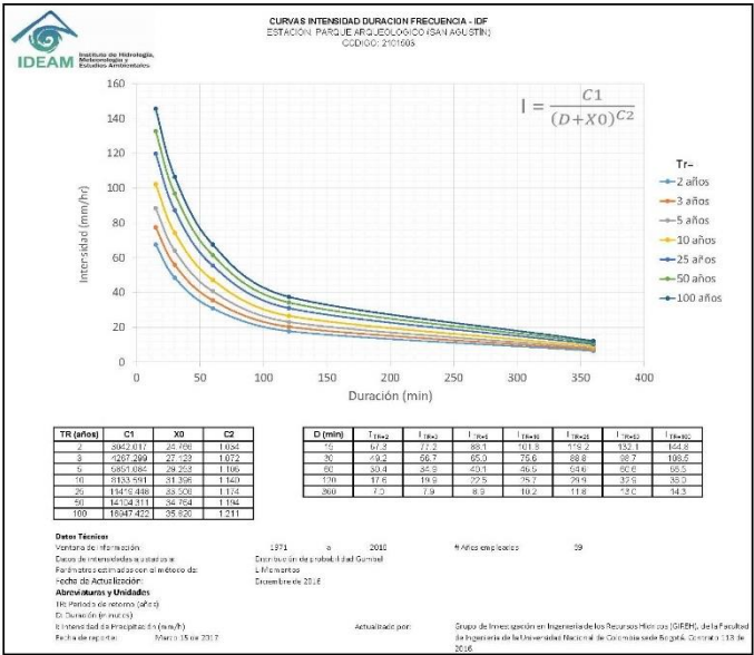
Gráfico 12. CURVAS IDF
