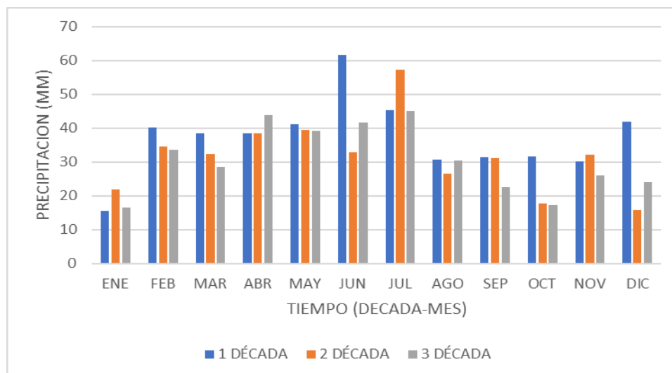
Gráfico 4. Promedios mensuales multianuales de precipitación de la estación Sevilla
