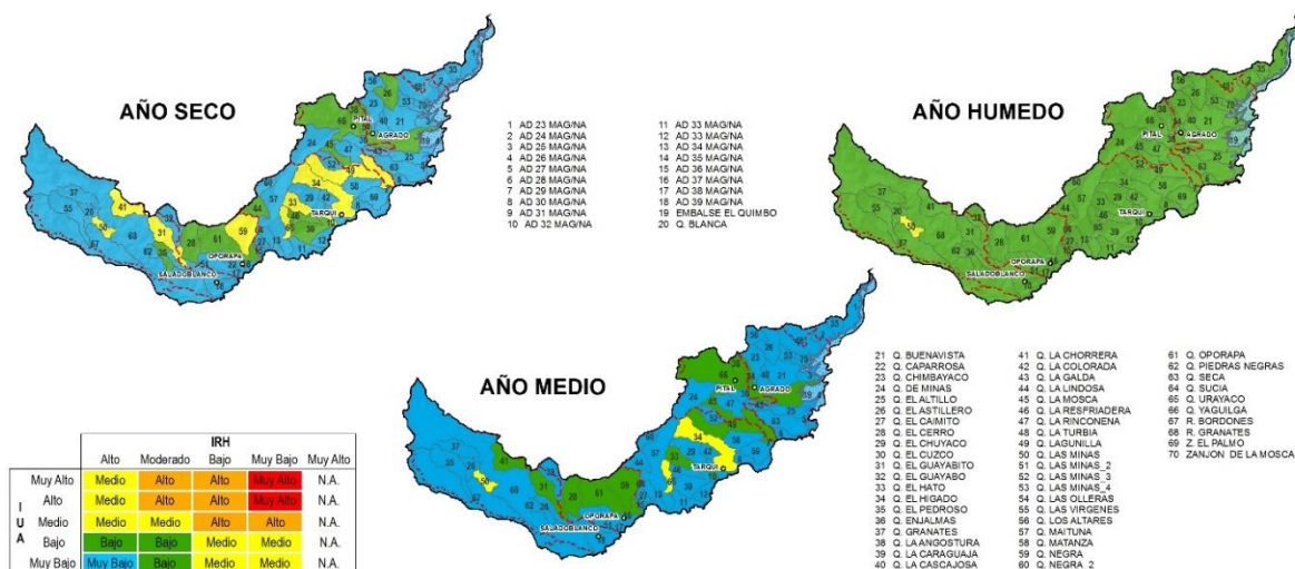
Figura 17. Índice de vulnerabilidad por desabastecimiento hídrico (IVH) SZH 2104 – Ríos Directos al Magdalena (mi).
