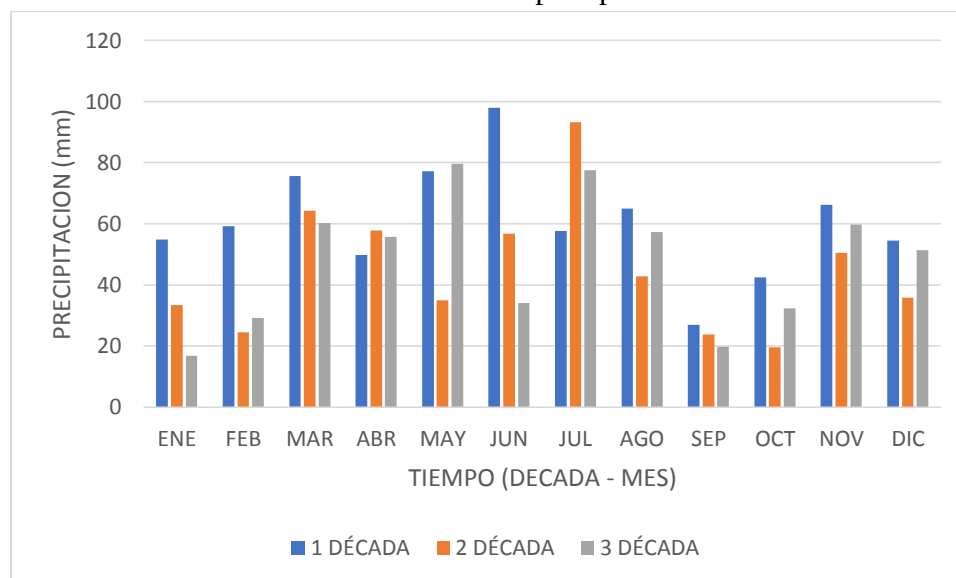
Gráfico 5. Promedios mensuales multianuales de precipitación de la estación El Dorado
