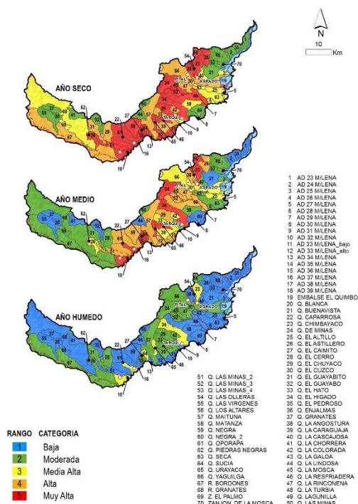
Figura 16. Índice de alteración potencial de la (IACAL) SZH 2104 – Ríos Directos al Magdalena (mi).
