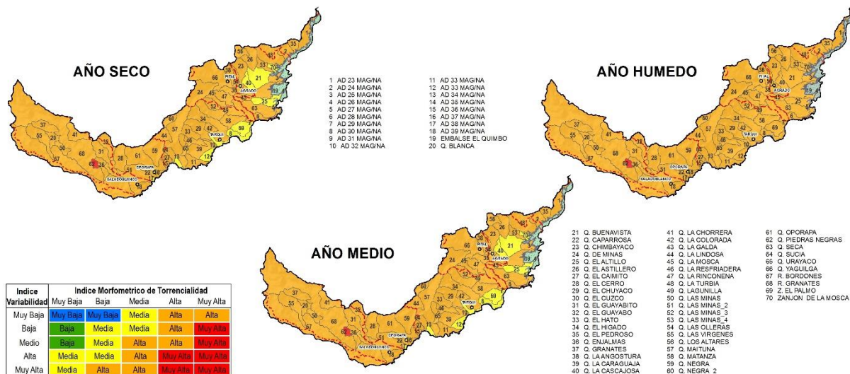
Figura 18. Índice de vulnerabilidad a eventos torrenciales (IVET) SZH 2104 – Ríos Directos al Magdalena (mi).
