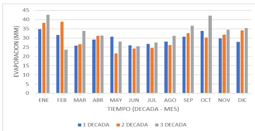
Gráfico 9. Valores medios decadales y mensuales multianuales de Evaporación de la estación Sevilla
