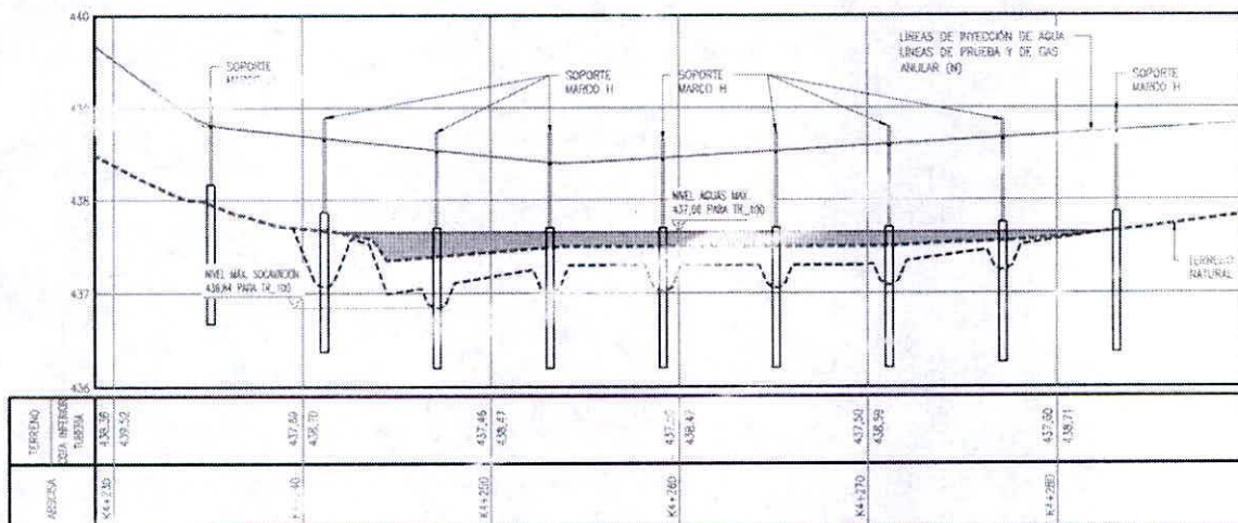
Perfil cruce P7
