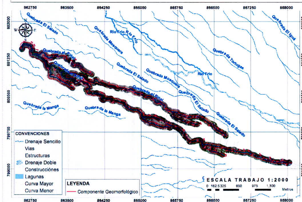
MAPA 9 - COMPONENTE GEOMORFOLÓGICO
