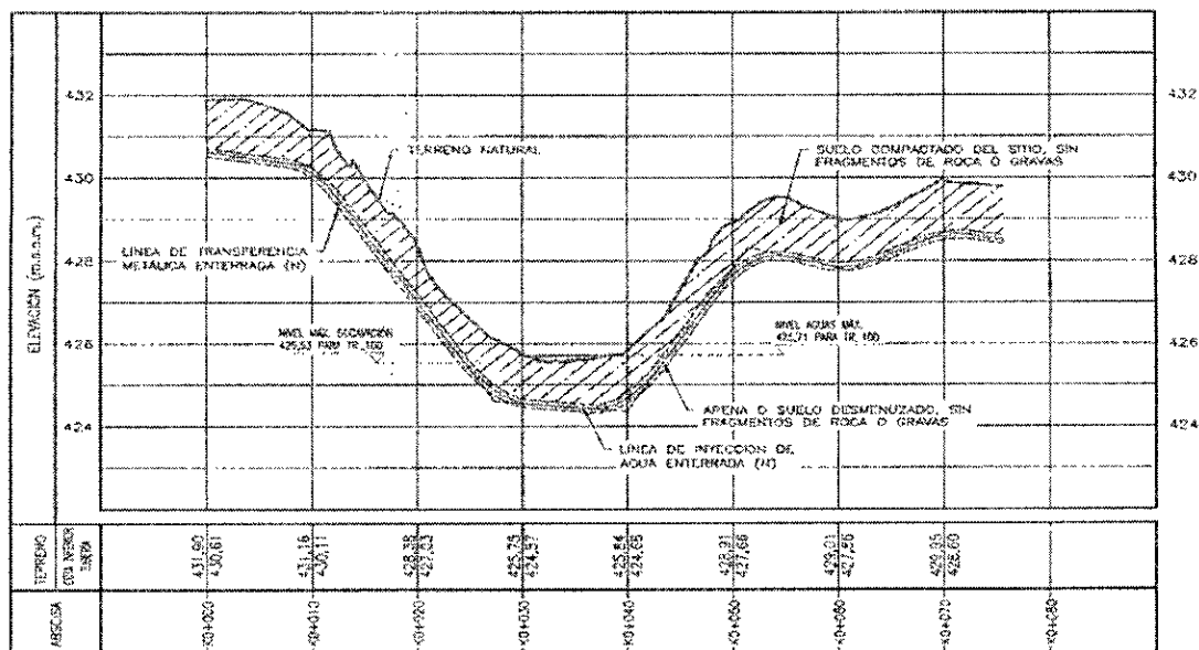
CRUCE D1 DETALLE PERFIL ESCALA H 1:500 ESCALA V 1:100
