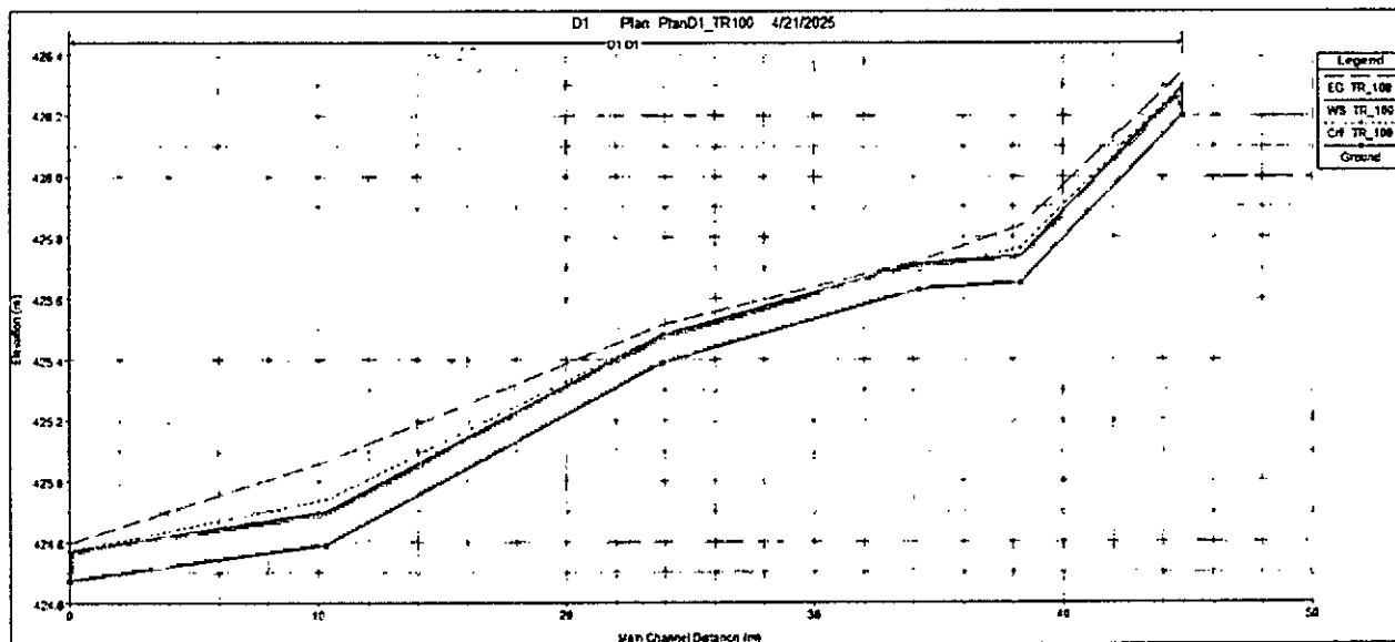
Figura 25. Perfil longitudinal del flujo para el periodo de retorno de 100 años – Cruce D1, condiciones existentes
