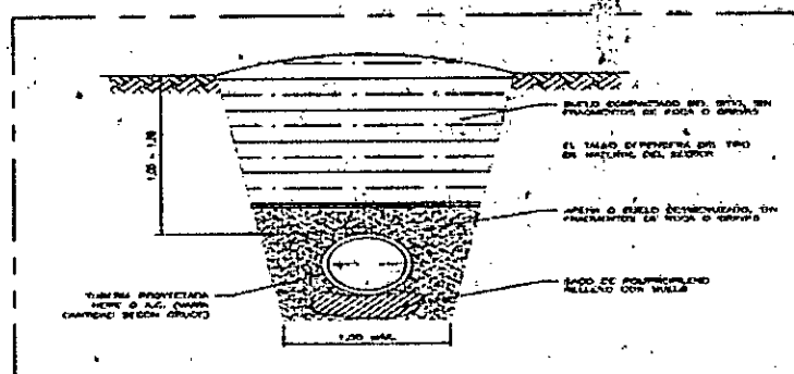
ZANJA TIPO PARA TUBERÍA ENTERRADA CON ESCALA
