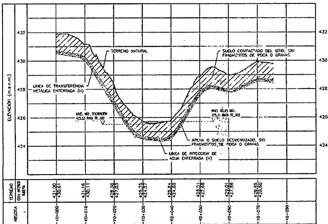
CRUCE D1 DETALLE PERFIL
