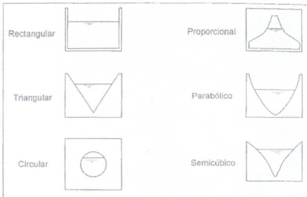
Figura 1 Formas de vertedero
