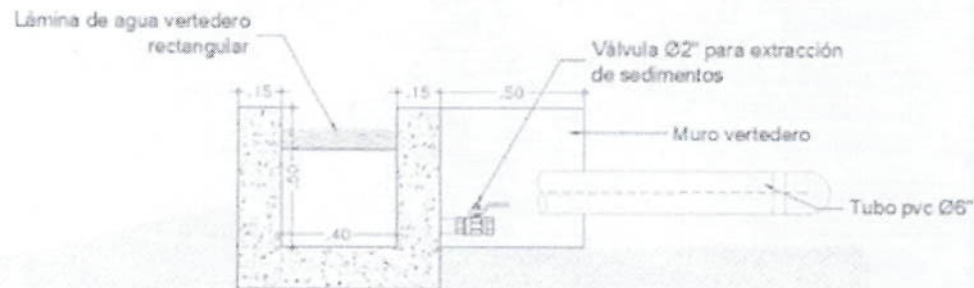
Figura 9 Obra de Control Vista Frontal
