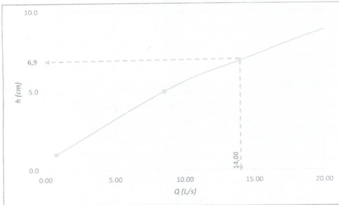
Figura 7 Altura lámina de agua vs caudal
