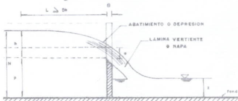
Figura 6 Localización Limnómetro
