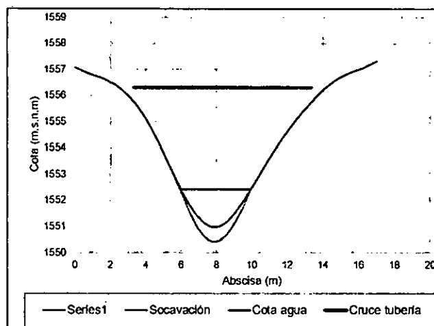
Imagen 8. Figura 7-1. Socavación general en condiciones existentes para la quebrada Mercedes (K0+220,05)
