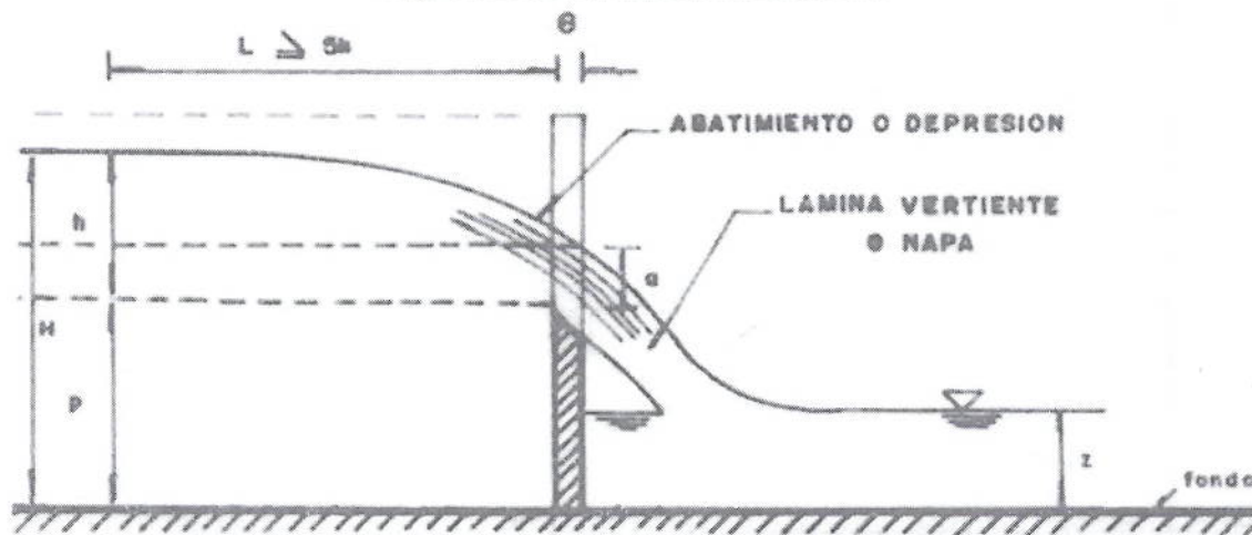
Figura 9 Localización Limnómetro
