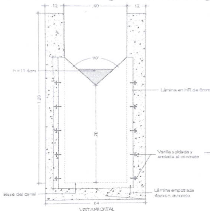
Figura 7 Vertedero Triangular de Pared Delgada
