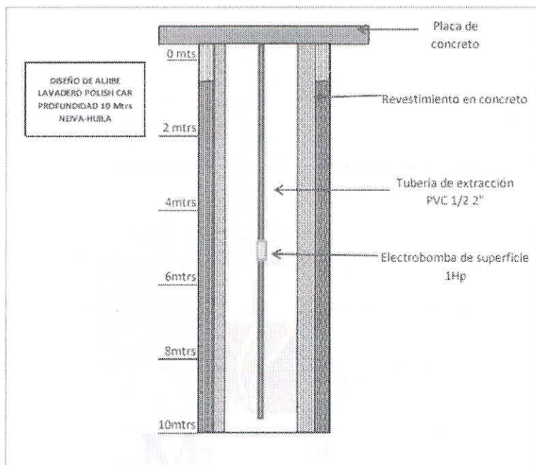
Imagen 11. Diseño del aljibe objeto a concesionar. Fuente. Informe técnico – Prueba de bombeo para determinación de parámetros hidráulicos e hidrogeológicos, presentado por el interesado.
