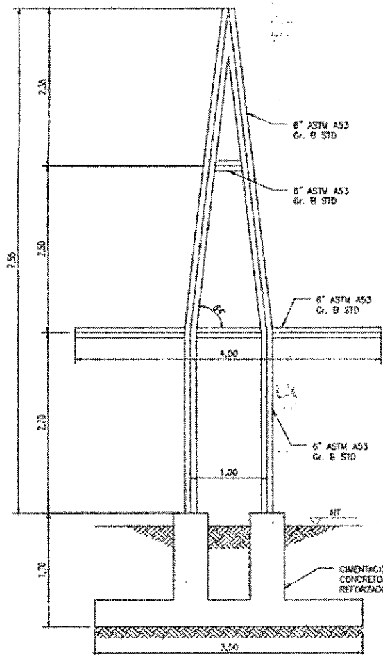
ALZADO TORRE — 1 DIMENSIONES ESCALA 1:50
