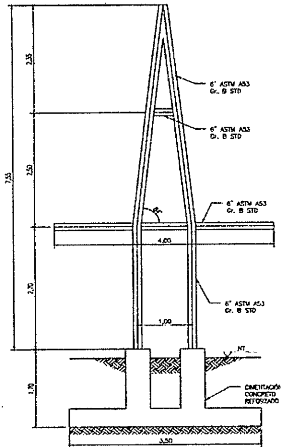
ALZADO TORRE - 1 DIMENSIONES ESCALA 1:50
