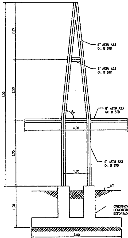
ALZADO TORRE - 1 DIMENSIONES ESCALA 1:50
