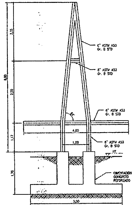
ALZADO TORRE - 2 DIMENSIONES ESCALA 1:50
