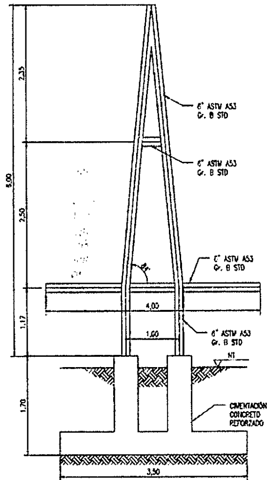
ALZADO TORRE - 2 DIMENSIONES ESCALA 1:50
