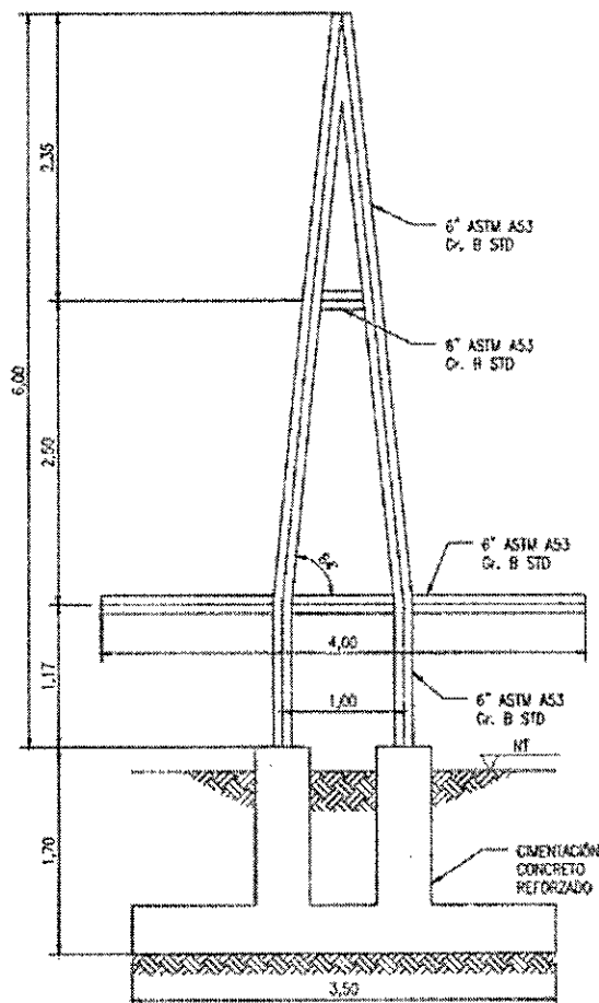
ALZADO TORRE — 2 DIMENSIONES ESCALA 1:50
