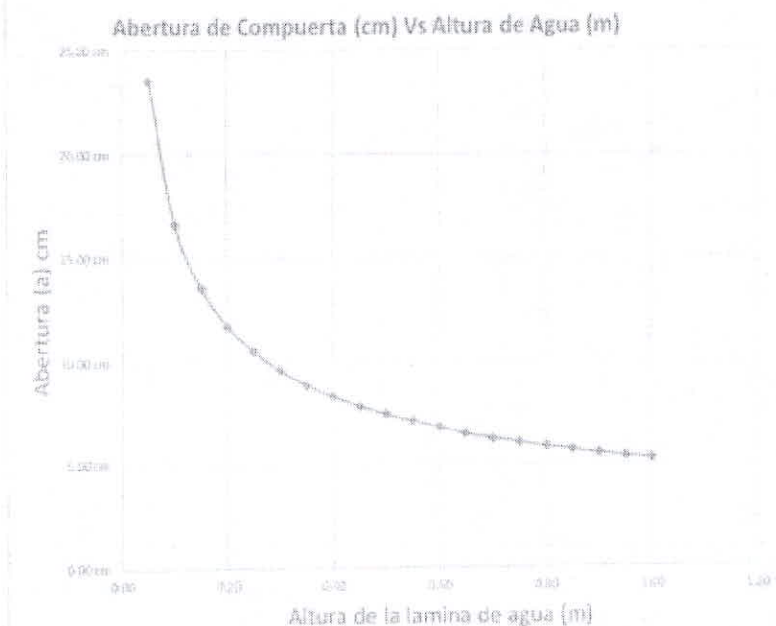
Ilustración 13. diseño de los valores obtenidos para la medición de caudales en verano por medio de una regleta graduada. Fuente: Radicado CAM-18958
