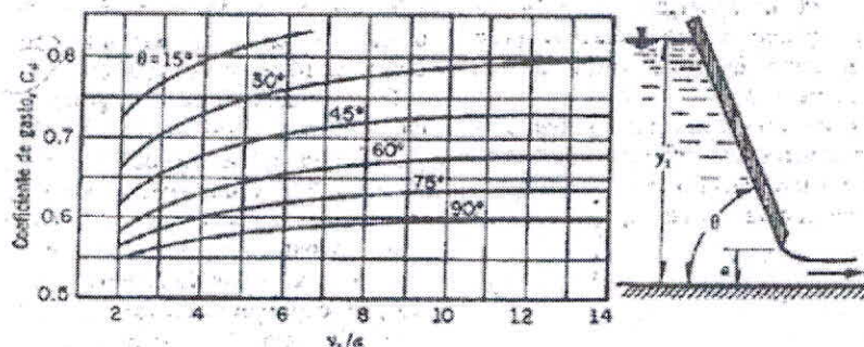
Ilustración 9. Coeficiente de gastos para compuertas planas inclinadas con descarga libre. Fuente: Radicado CAM-18958 planas obtenidos con un ángulo de inclinación \theta en términos de la ecuación y_1/a .
