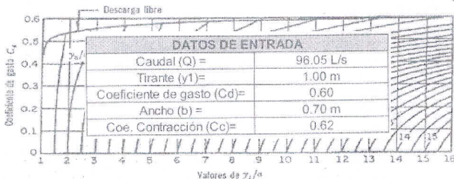
Ilustración 10. Coeficientes de gasto para compuertas planas e inclinadas con descarga libre. Fuente: Radicado CAM-18958 A continuación, se presenta la tabla resumen de los cálculos realizados para la obtención de los resultados de diseño del caudal de verano ( v ) para la compuerta plana deslizante.
