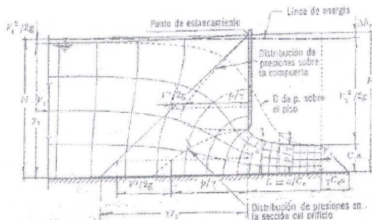
Ilustración 8. Red de flujo para una compuerta plana (deslizante). Fuente: Radicado CAM-18958
