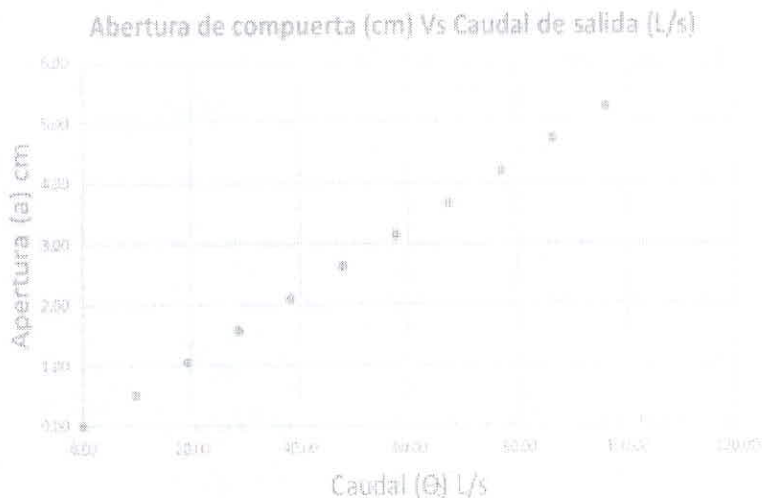
Ilustración 12. Curva de calibración apertura vs cauda en veranol. Fuente: Radicado CAM-18958 caudal (l/s)
