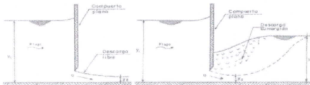
Ilustración 7. Tipo de descarga en compuertas. Fuente: Radicado CAM-18958
