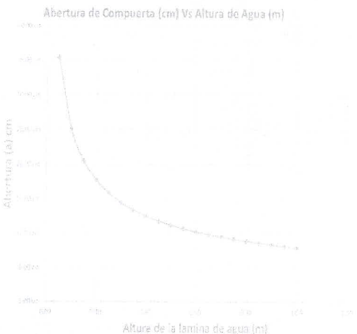
Ilustración 16. diseño de los valores obtenidos para la medición de caudales en invierno por medio de una regleta graduada. Fuente: Radicado CAM-18958
