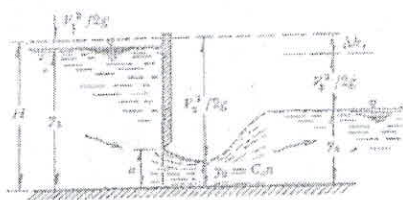
Ilustración 6. Detalle de compuerta deslizante. Fuente: Radicado CAM-18958
