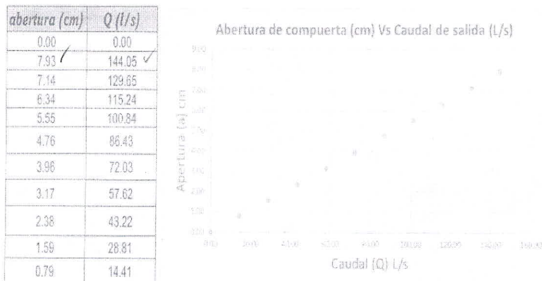
Ilustración 15. Curva de calibración abertura vs caudal en invierno. Fuente: Radicado CAM-18958
