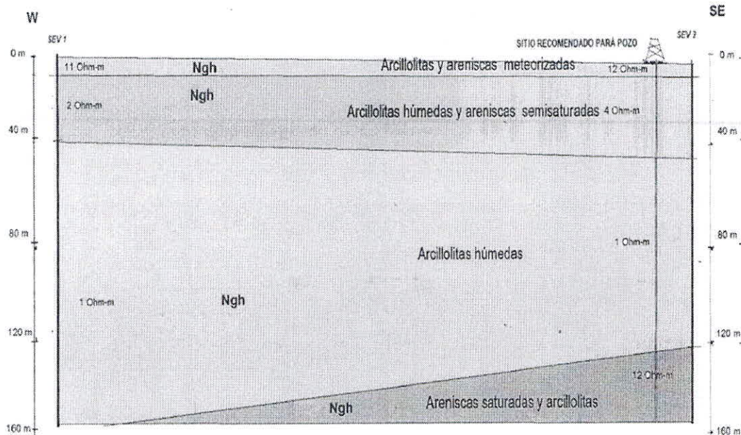
Imagen 5. Perfil geoelectrico de la zona presentado en el "ESTUDIO GEOELECTRICO PARA LA DETERMINACION DE LA UBICACIÓN DE UN POZO EXPLORATORIO PARA AGUA SUBTERRANEA PARA LA VEREDA DINDAL, CRUCE GUACIRCO, MUNICIPIO DE AIPE (HUILA)"
