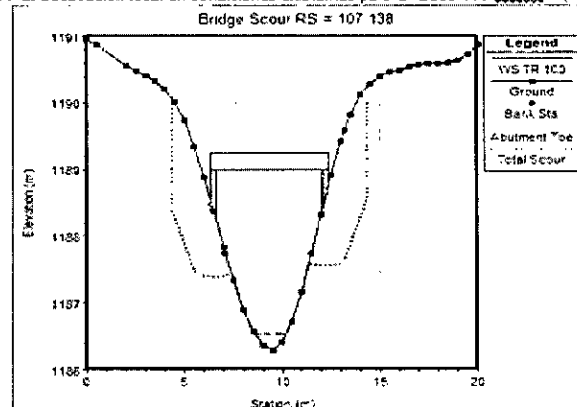
Figura 7-2. Socavación local en condiciones existentes para El Quebrada Libano 1 (KD+182.00)
