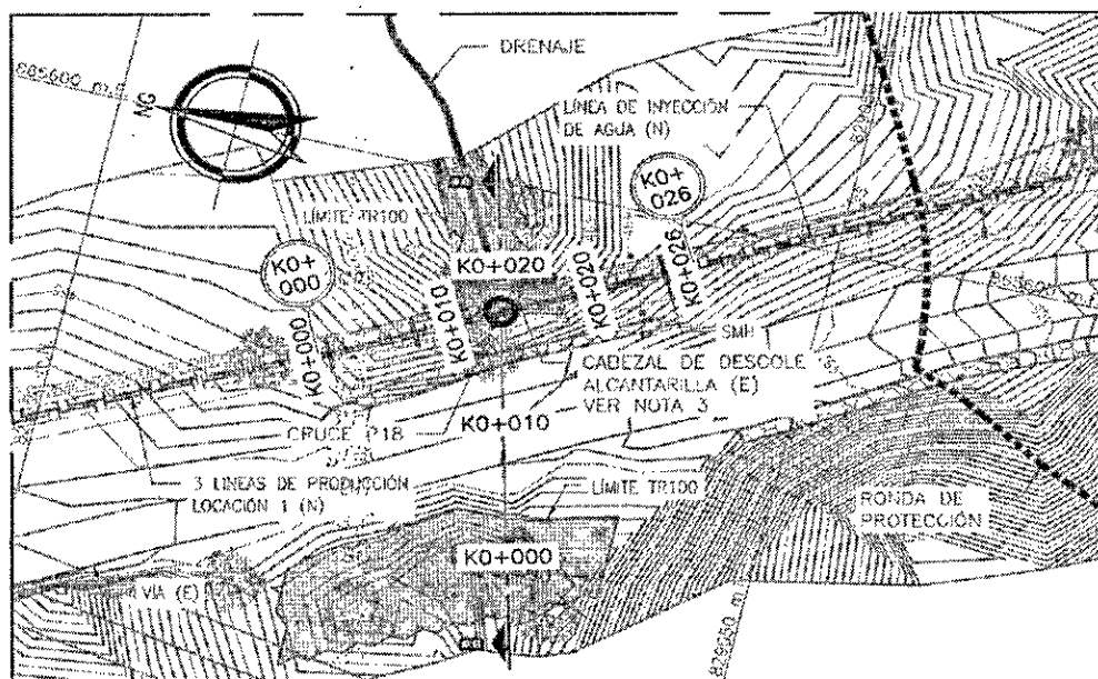
Planta de localización cruce P18
