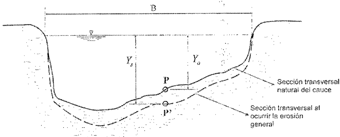
Figura 1. Esquema de descenso del lecho por socavación general.
