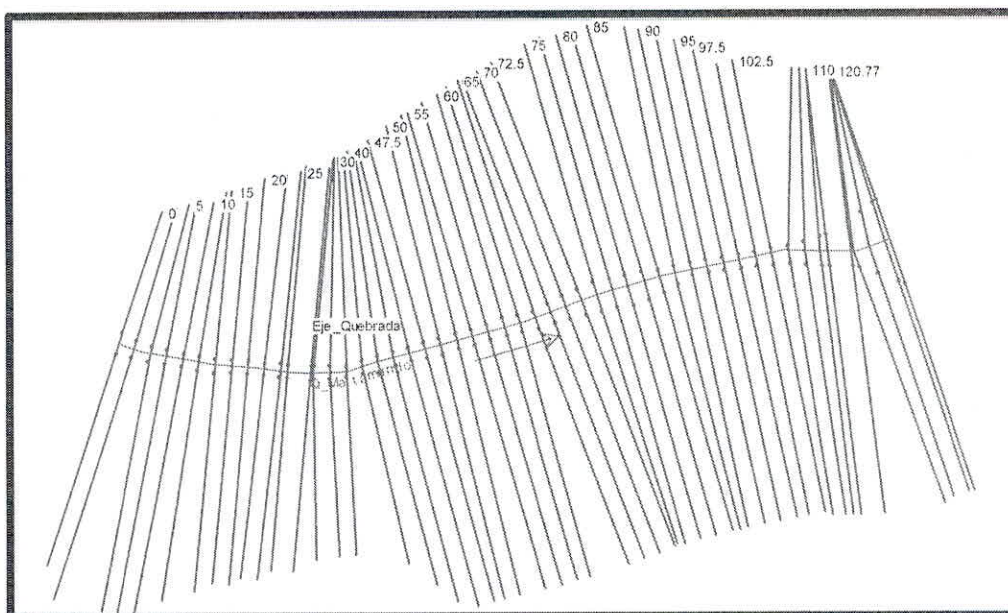
Imagen 2. Figura 1. Geometría de la superficie del cauce de la Quebrada Matamundo y secciones de trabajo.
