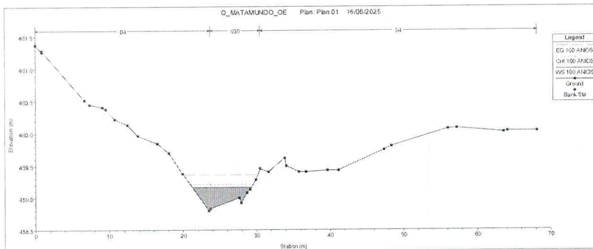
Imagen 3. FIGURA 3. Resultado grafico de la simulación hidráulica de la Quebrada Matamundo en la estación 114.68. Aguas arriba Puente 2.
