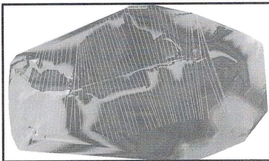
Imagen 8. FIGURA 8. Resultado grafico de la simulación hidráulica de la Quebrada Matamundo
