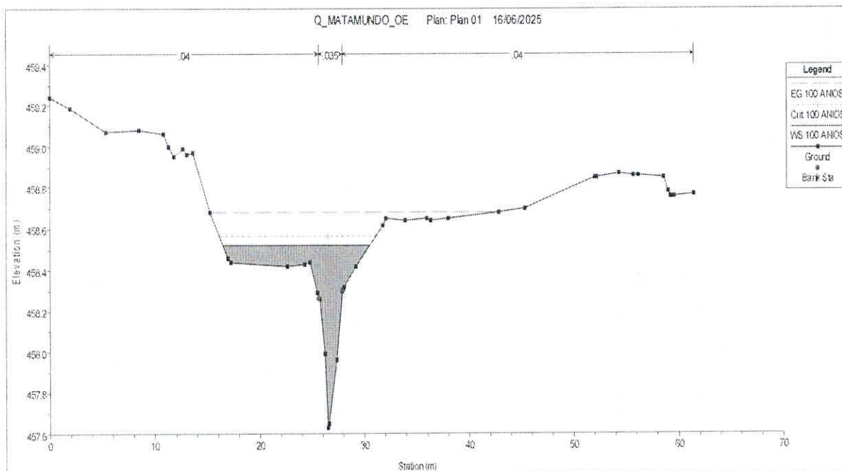
Imagen 7. FIGURA 7. Resultado grafico de la simulación hidráulica de la Quebrada Matamundo en la estación 0.
