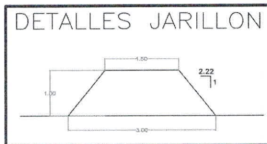
Imagen 10. FIGURA 10. Dimensiones del jarillon propuesto
