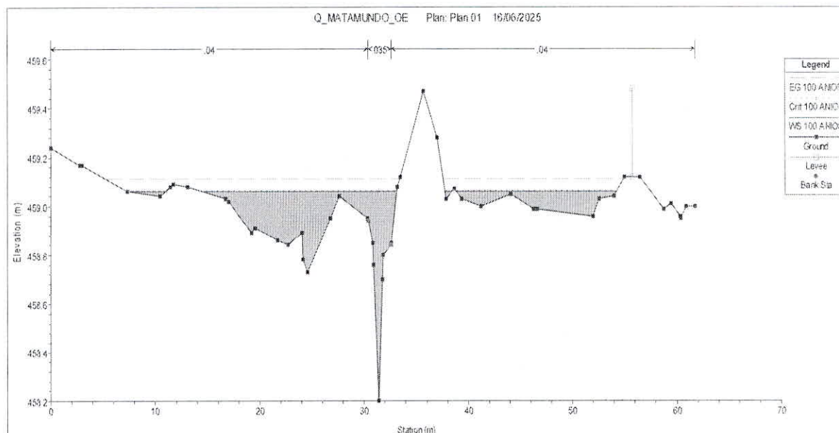
Imagen 5. FIGURA 5. Resultado grafico de la simulación hidráulica de la Quebrada Matamundo en la estación 29.63. Aguas arriba Puente 1.
