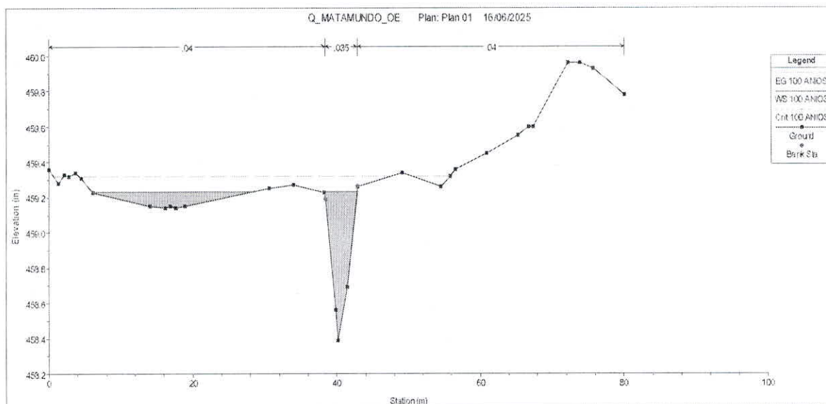
Imagen 4. FIGURA 4. Resultado grafico de la simulación hidráulica de la Quebrada Matamundo en la estación 77.5.
