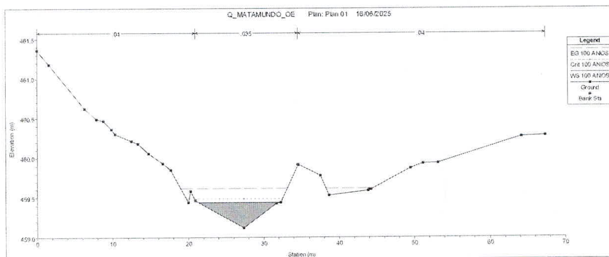
FIGURA 2. Resultado grafico de la simulación hidráulica de la Quebrada Matamundo en la estación 120.77
