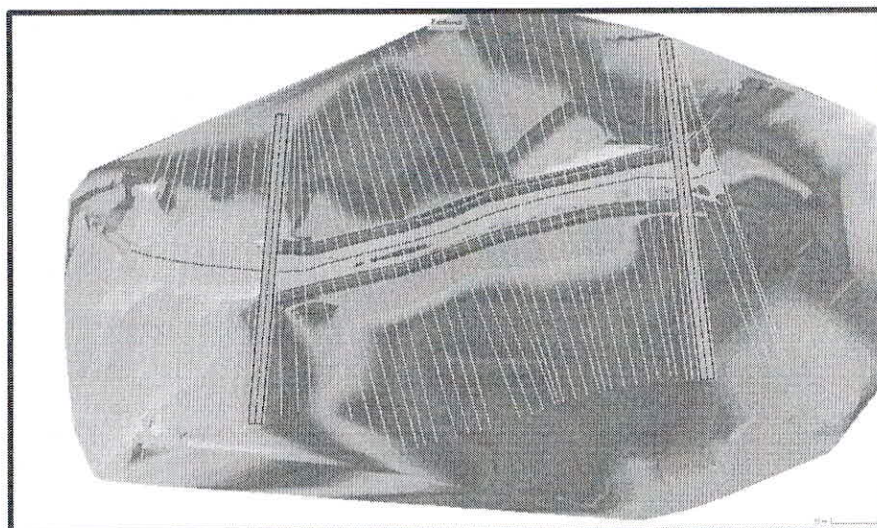
Imagen 14 .FIGURA 14. Resultado grafico de la simulación hidráulica de la Quebrada Matamundo con obra implantada
