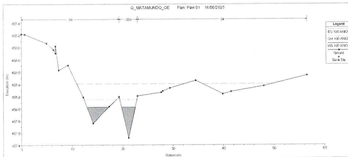
Imagen 7. FIGURA 7. Resultado grafico de la simulación hidráulica de la Quebrada Matamundo en la estación 0.
