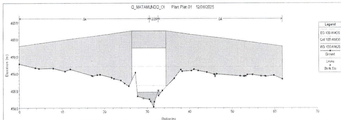
Imagen 12. FIGURA 12. Resultado grafico de la simulación hidráulica del puente 1 en la estación 27.87 aguas arriba.
