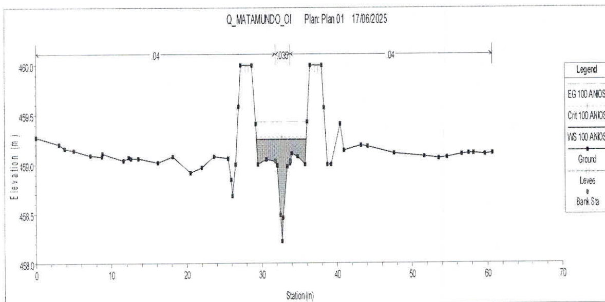
Imagen 13 .FIGURA 13. Resultado grafico de la simulación hidráulica del jarillón en la estación 32.5.
