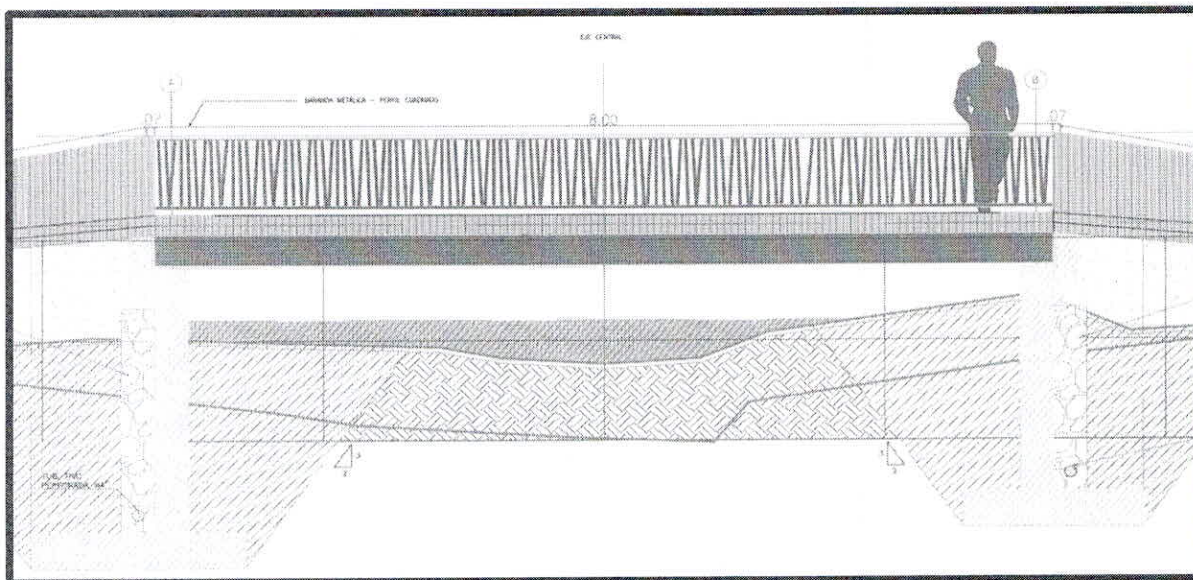
Imagen 9. FIGURA 9. Dimensiones de puente peatonal "Puente 1".
