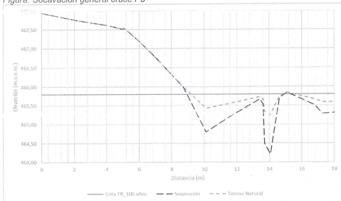
Figura. Socavación general cruce P5
