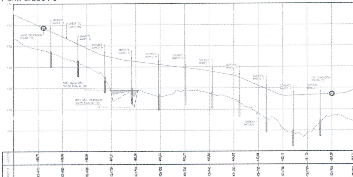
Perfil cruce P5
