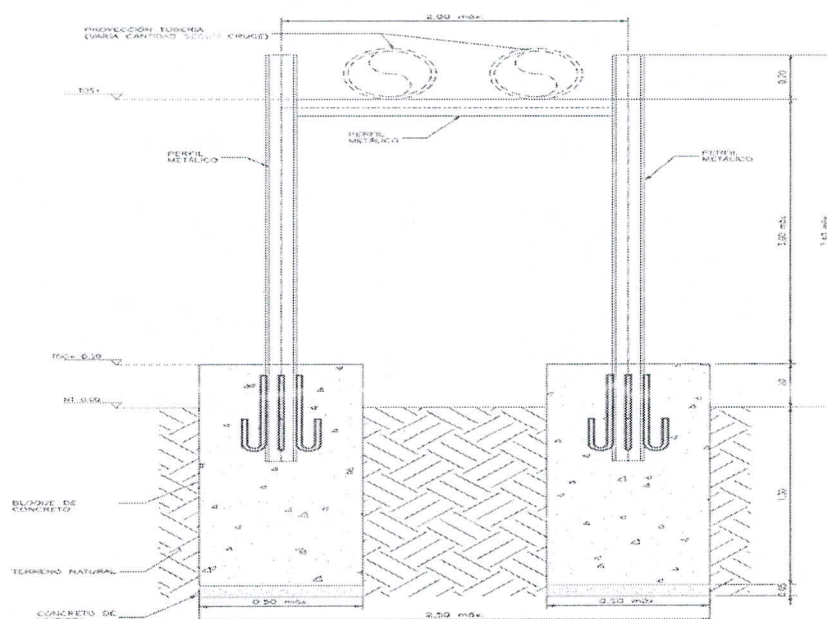
Estructura definida cruce menor P5
