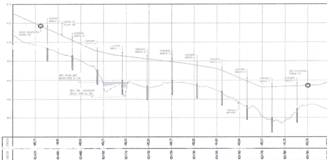
Perfil cruce P5
