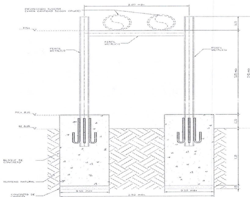
Estructura definida cruce menor P5
